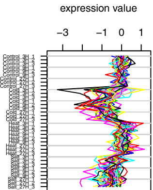
Cluster 9 ( 42 genes )
