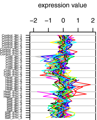
Cluster 8 ( 61 genes )
