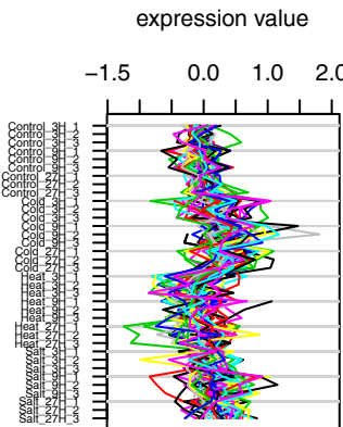
Cluster 5 ( 54 genes )
