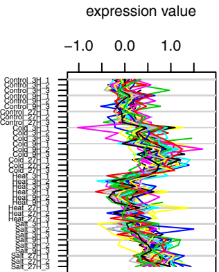
Cluster 7 ( 35 genes )
