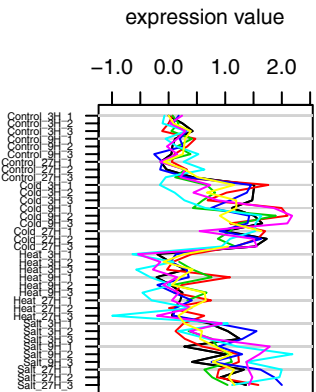
Cluster 6 ( 7 genes )
