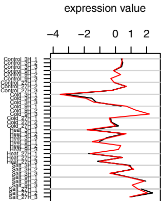
Cluster 4 ( 2 genes )
