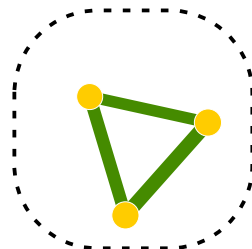
module8 (p.value=5.14e-03)
