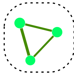
module8 (p.value=5.14e-03)
