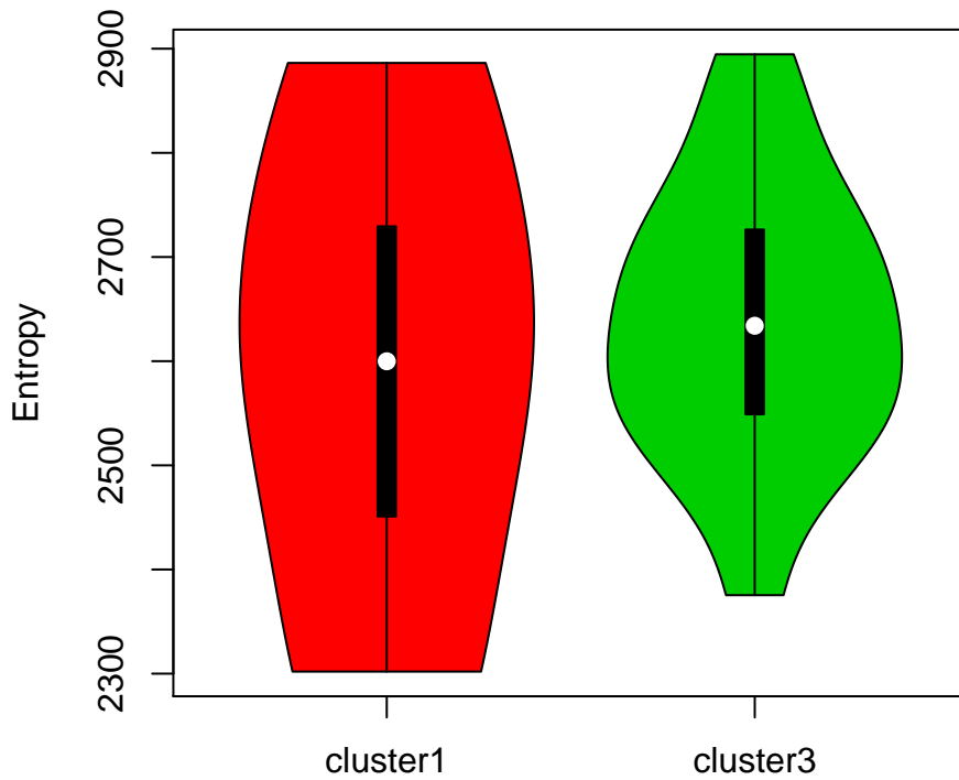
Cluster Entropies
